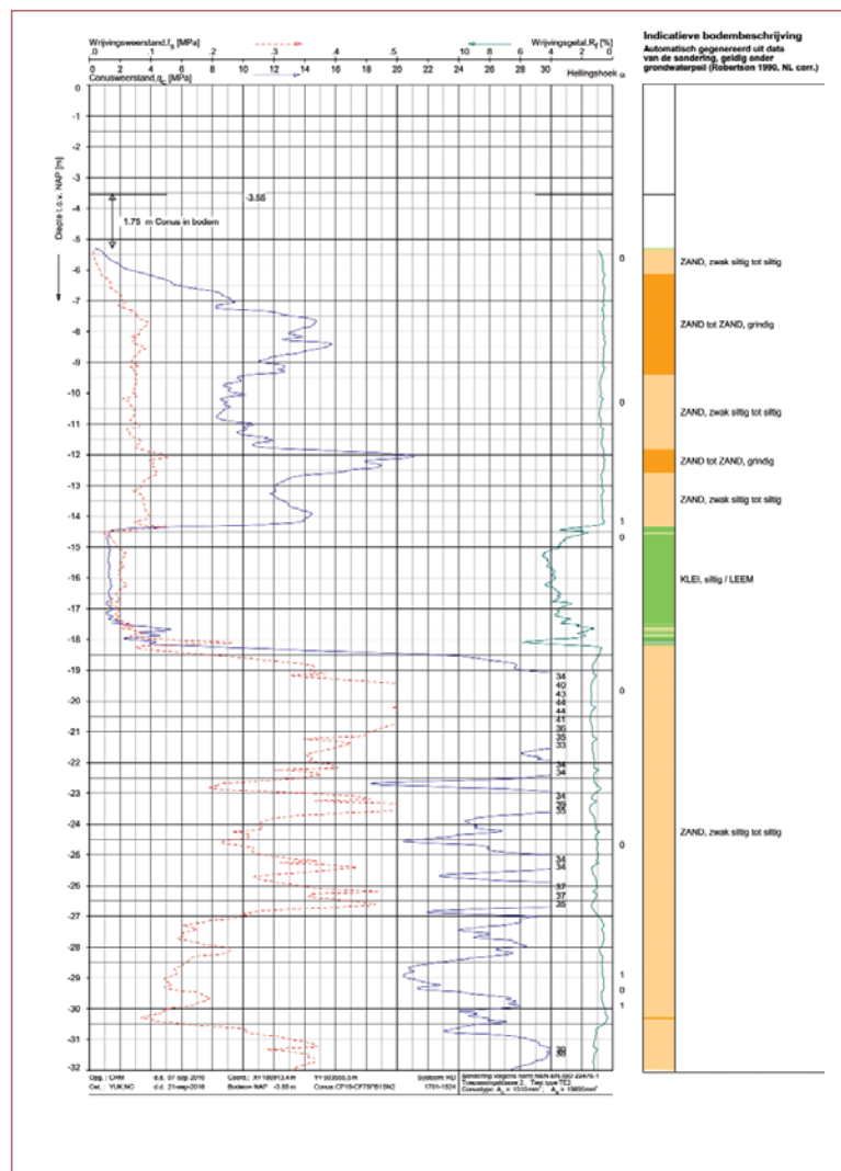
Figuur 4 – Representatieve sondering Reeve- sluiscomplex.
